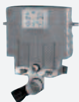
38 415 Uniset modulo per vaso sospeso cassetta di sciacquo GD2, 6-9 l valvola di scarico AV1 con 3 tipi di azionamento dual flush, start/stop e un solo sciacquo altezza di installazione 0,82, azionamento frontale o dall'alto custodia insonorizzata in EPS per il rivestimento in muratura
